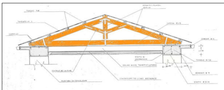
capriata lignea ed interni di S. Anna
