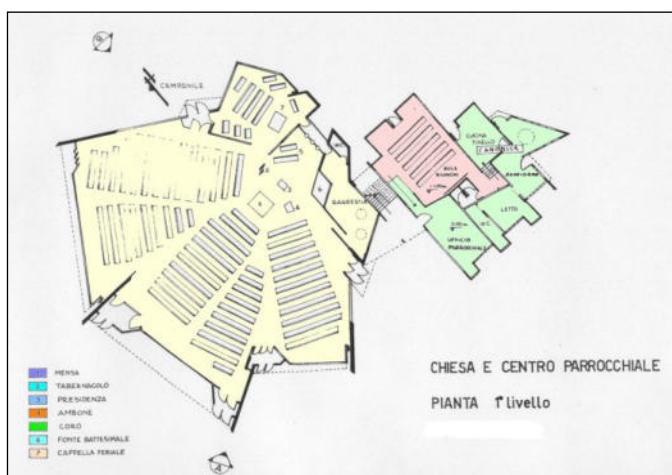
Pianta del nuovo complesso religioso e schizzo della vista dell'interno della chiesa
