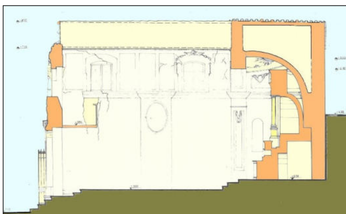
capriata lignea ed interni di S. Anna
