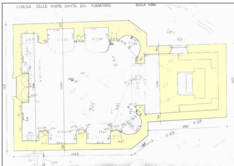
pianta della Chiesa del purgatorio schizzi del rilievo
