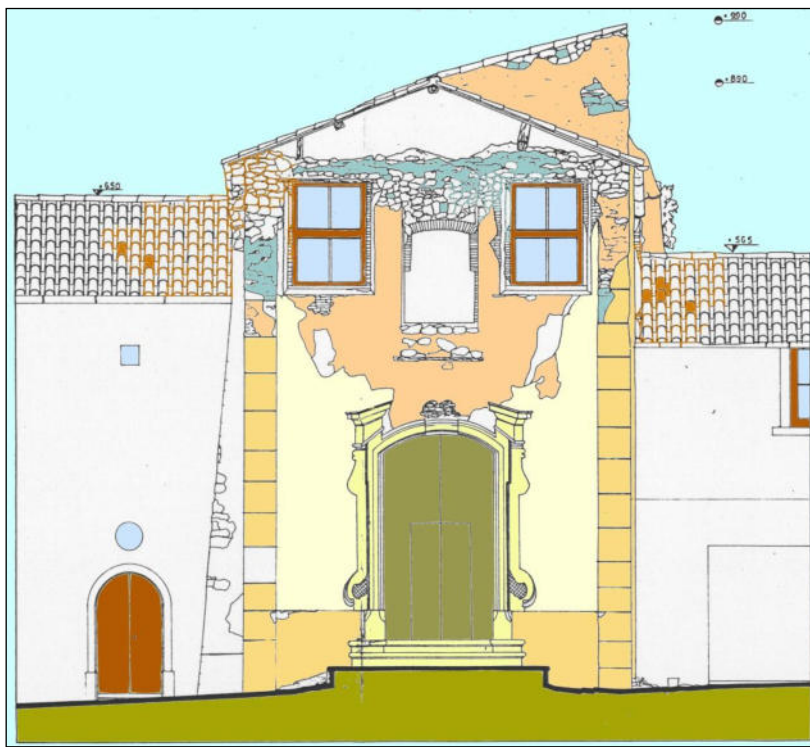
prospetto di S. Anna
